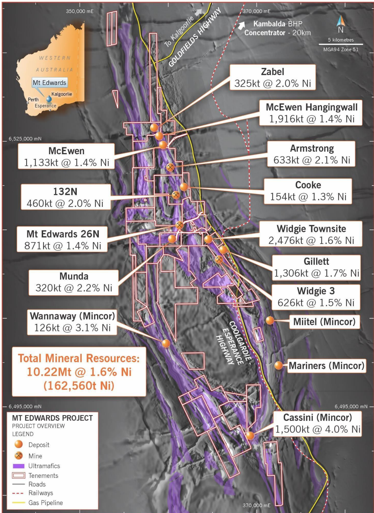
Abbildung 1 - Bergbau-Tenements des Mt. Edwards-Projekts über Geologie.
